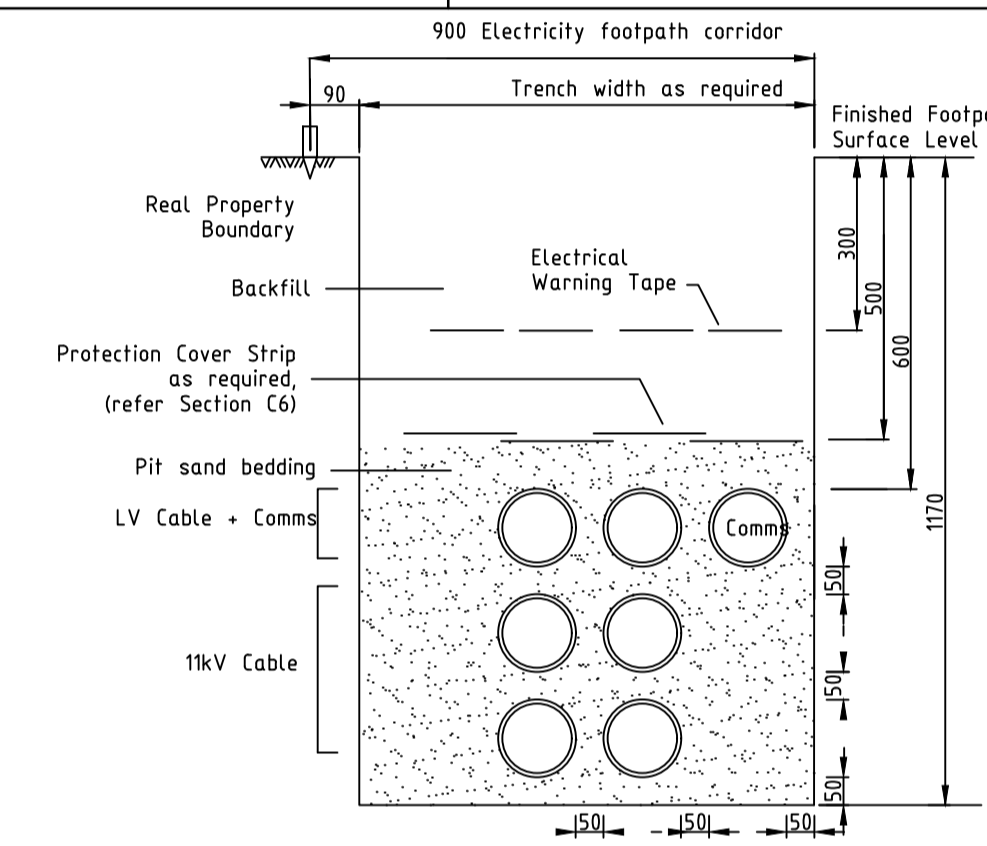
11kV NETWORK
